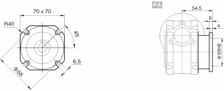
Output flange 输出法兰
